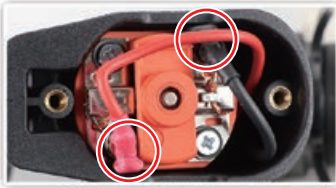
無作動 檢查馬達連接線(需卸下底板)。
