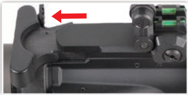
Halando la manija de carga llevará el cerrojo atrás y abrirá la cubierta.
